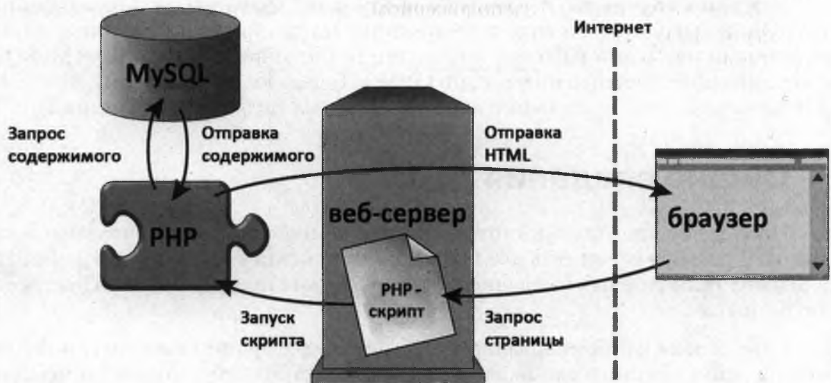
Рис. 4.1. PHP извлекает данные из MySQL для создания веб-страниц
