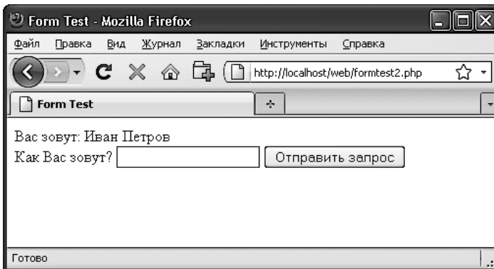
Рис. 11.2. Программа formtest.php с обработкой данных
