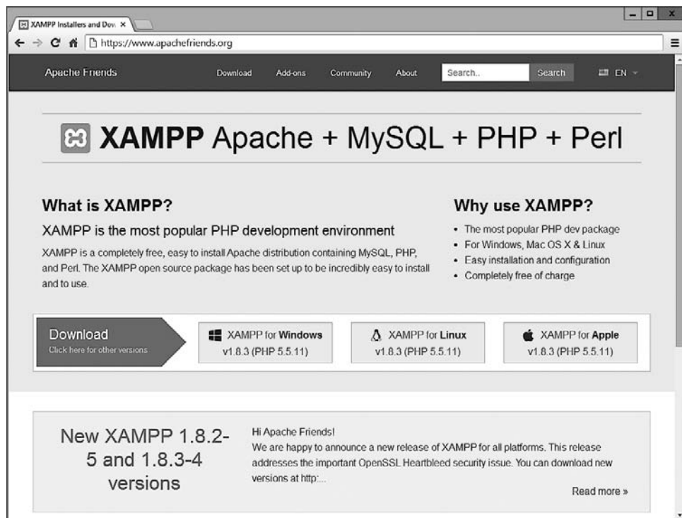
Рис. 2.1. Сайт XAMPP
