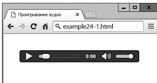
Рис. 24.1. Проигрывание аудиофайла
