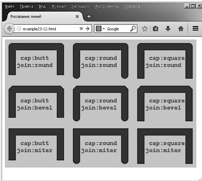
Рис. 23.11. Все комбинации законцовок и соединений линий
