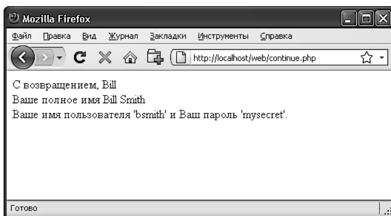
Рис. 12.5. Поддержка пользовательских данных с помощью сессий
