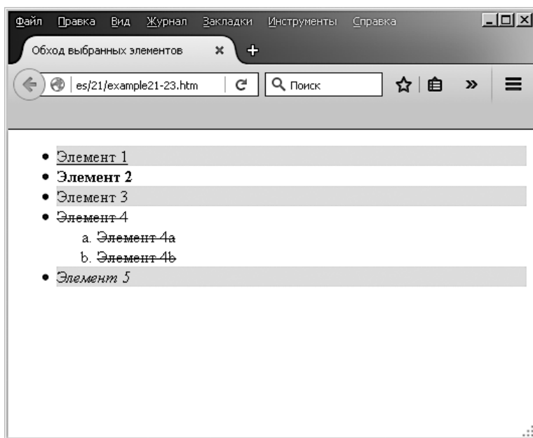
Рис. 21.21. Конкретная адресация элементов из тех, что были выбраны методами jQuery
