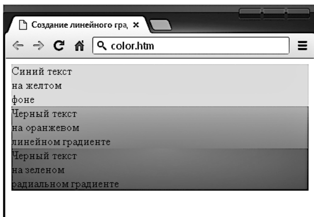
Рис. 18.10. Сплошной цвет фона, а также линейный и радиальный градиенты
