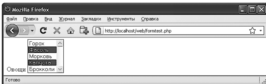
Рис. 11.7. Использование поля со списком с атрибутом multiple
