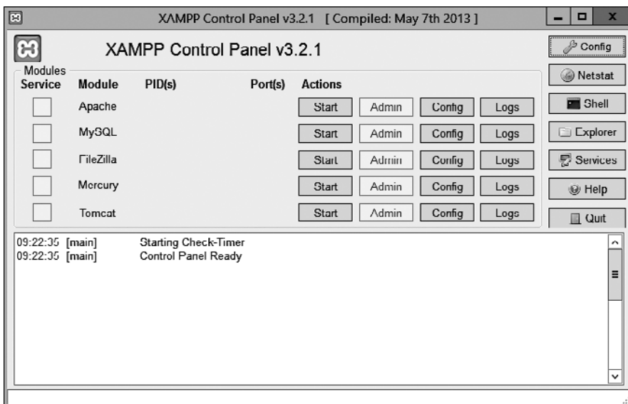
Рис. 2.9. Панель управления
